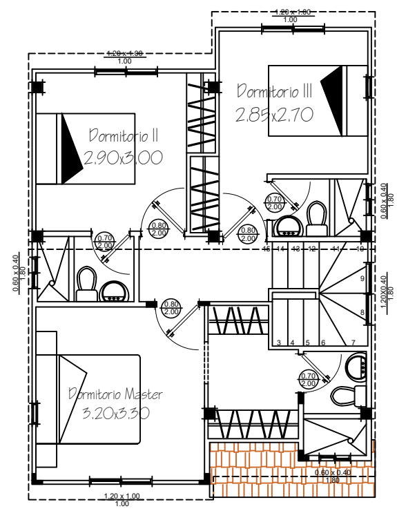
Planta Alta
