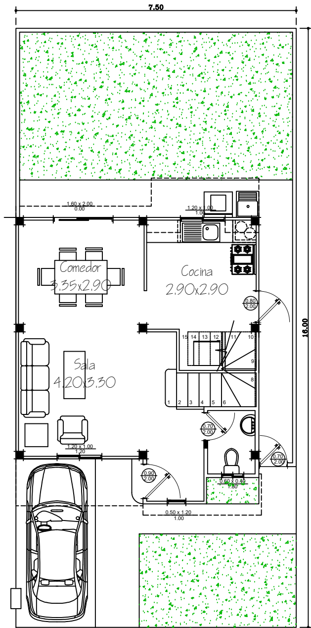
Planta Baja
