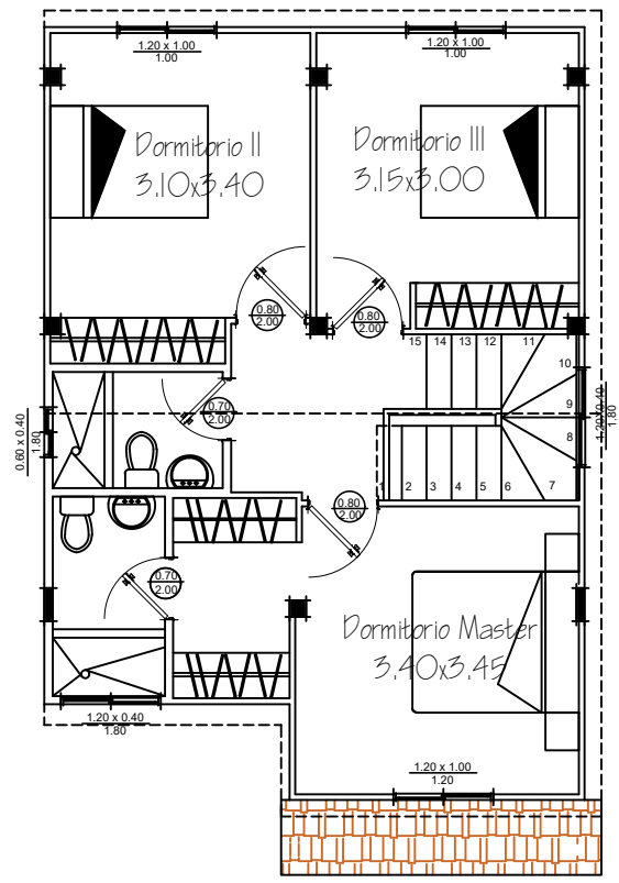
Planta Alta
